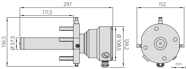
Abmessungen des PR53SD
