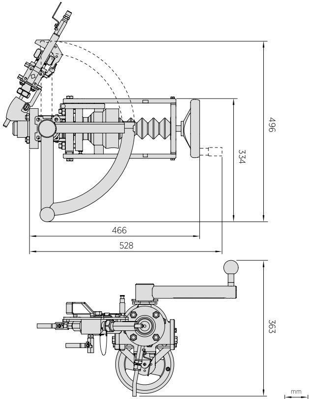
Abmessungen des PR53 SDI5 Safe-Drive Absperrventils und Retraktors
